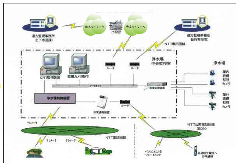
遠方監視システム
